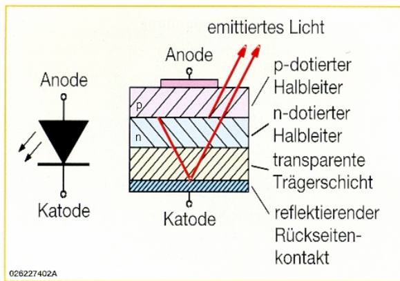
Bild 2: Prinzipieller Aufbau des Halbleiterkristalls einer LED
