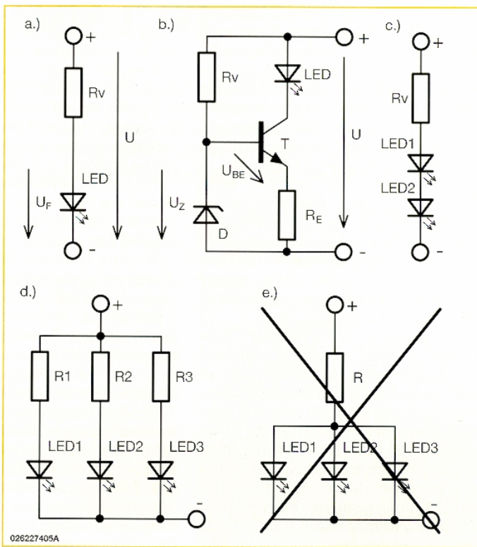
Bild 8: Schaltungsbeispiele für den Betrieb von LEDs
