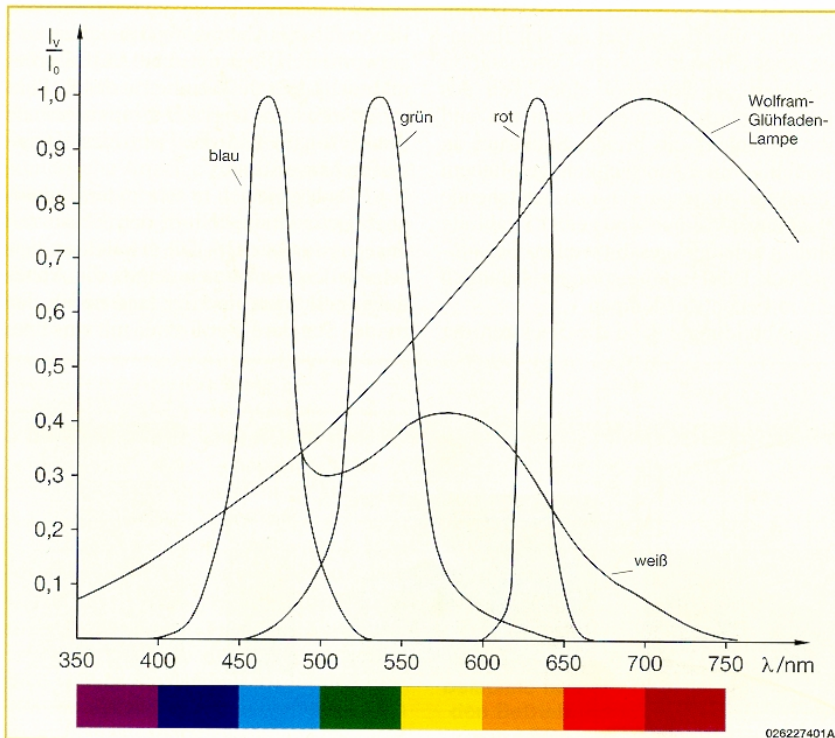
Bild 1: Spektrale Verteilung der Strahlung verschiedenfarbiger LEDs
