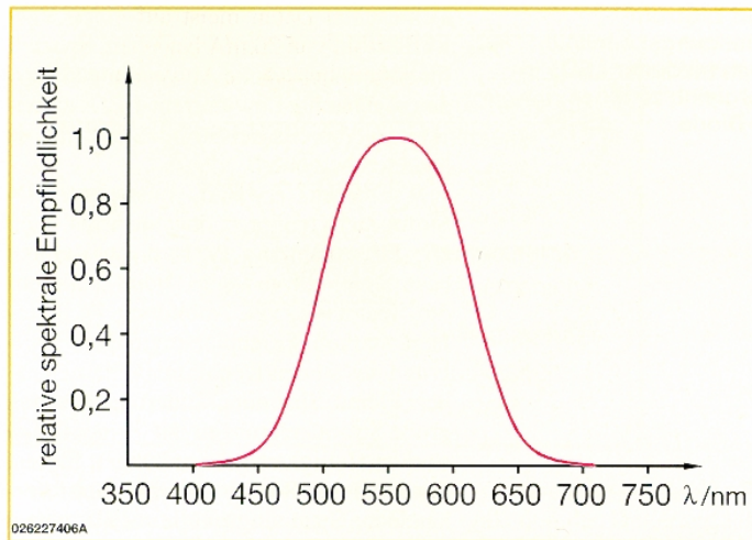
Bild 9: Spektrale Hellempfindlichkeit des menschlichen Auges (V(λ)-Kurve)
