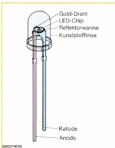
Bild 3: Prinzipieller Aufbau einer LED
